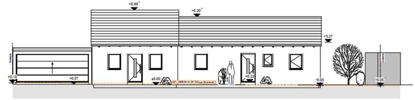
Ansichten Nord (Blumenstraße)
