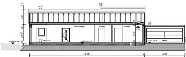
Schnitt B-B
